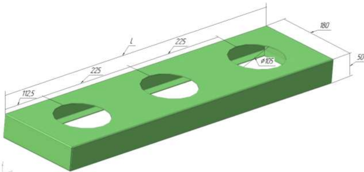
Рис.1 Подставка ДЖЕТ.608.00.00.00
