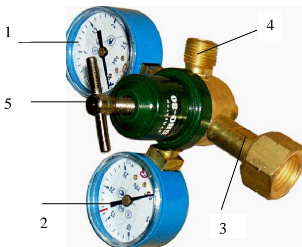
Рис.1 Редуктор БВО-80
