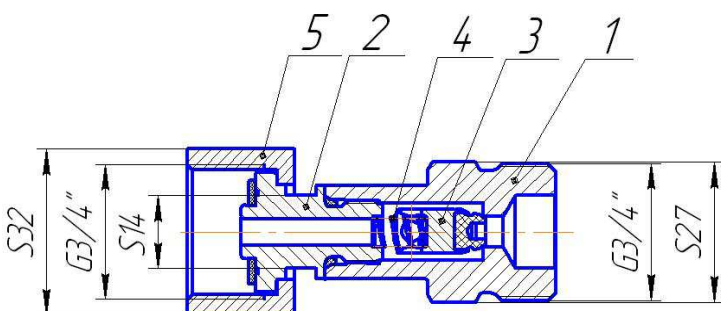
Рис.1 Клапан обратный ДЖЕТ 393 00 00 00
