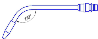
Рис.1 Горелка Г-2; Г-2У с наконечником ДЖЕТ 000 100 100-(01...11)
