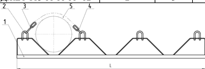
Рис.1 Ложемент рамповый ЛР ДЖЕТ 115 00 00 00
