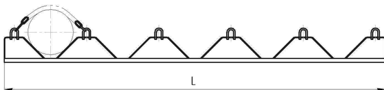
Рис.2 Ложемент рамповый ЛР ДЖЕТ 115 00 00 00-01
